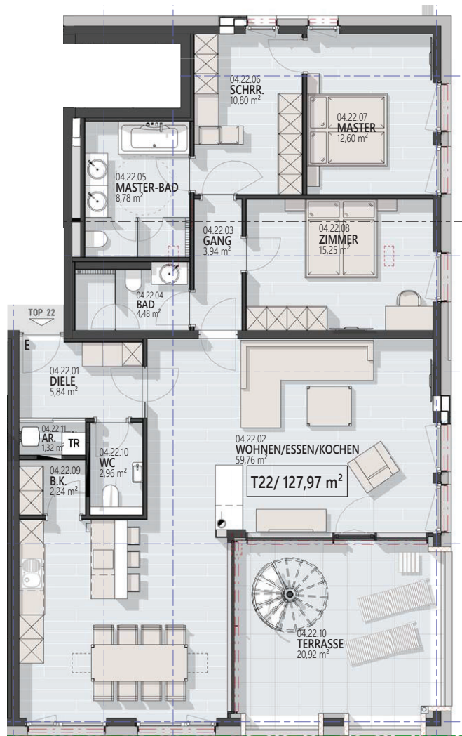
4. OG
